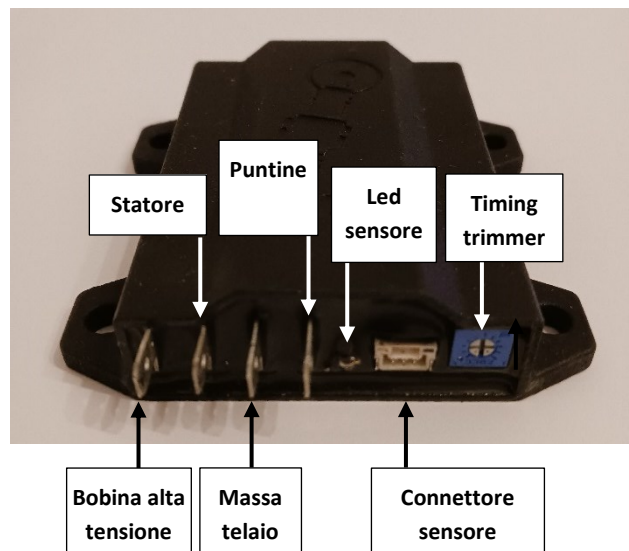
Figura 1: Vista frontale
