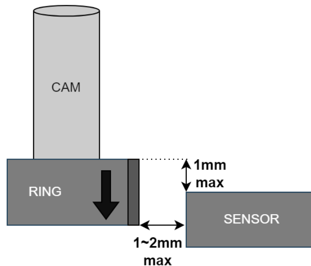
Figura 7: massima distanza e sfasamento tra sensore e anello
