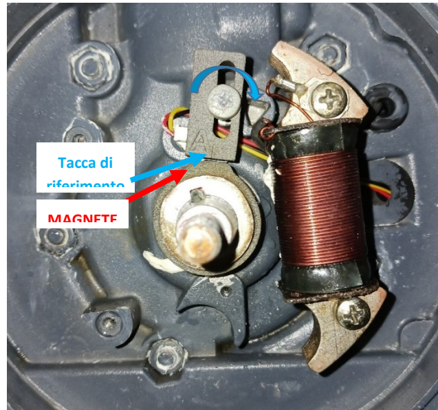
Figure 6: Montaggio sensore
